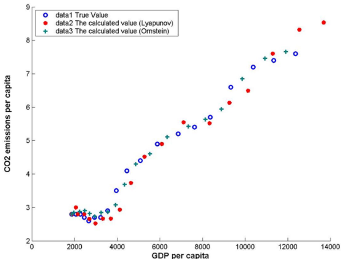
Рис. 3. Зависимость CO 2 эмиссии от GDP на душу населения в Китае за 1995–2013 гг. согласно натурным данным и рассчитанная методом Ляпунова и уравнением Орнштейна.
