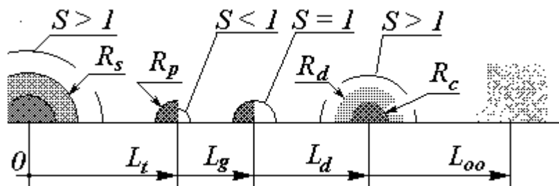
Рис. 1. Формирование диффузных планет Солнечной системы.
