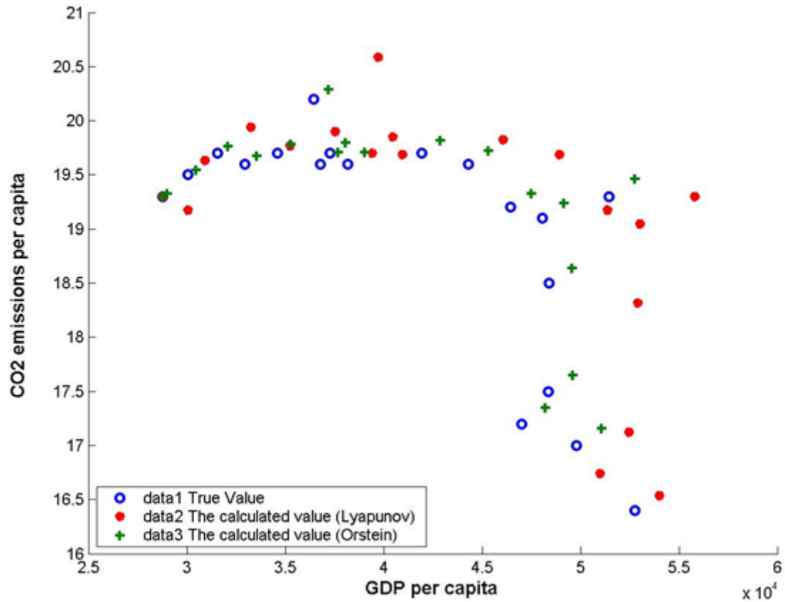
Рис. 2. Зависимость CO 2 эмиссии от GDP на душу населения в США за 1995–2013 гг. согласно натурным данным и рассчитанная методом Ляпунова и уравнением Орнштейна.
