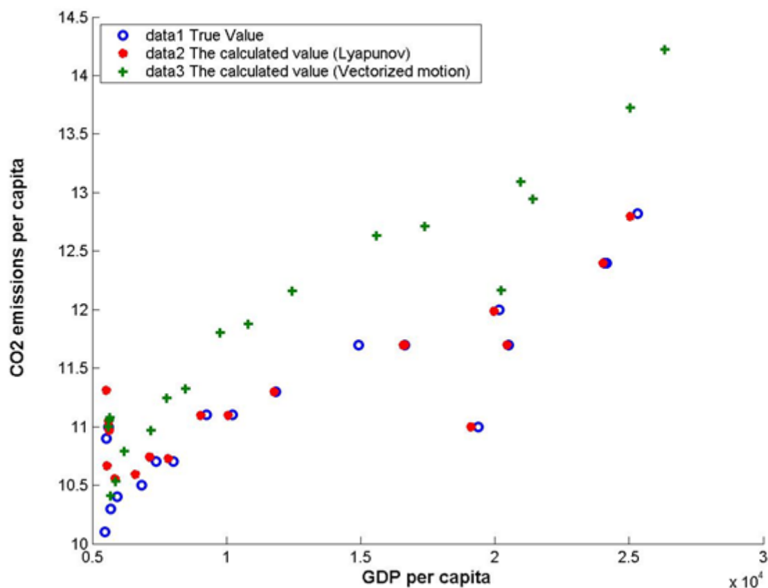
Рис. 1. Зависимость CO 2 эмиссии от GDP на душу населения в России за 1995–2013 гг. согласно натурным данным и рассчитанная методом Ляпунова и уравнением Эйнштейна-Смолуховского.
